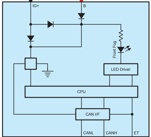
E22 Combination Meter
